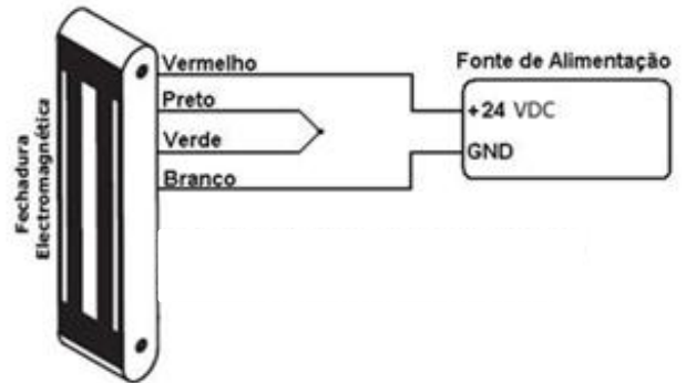
Conexão para 24 VDC
