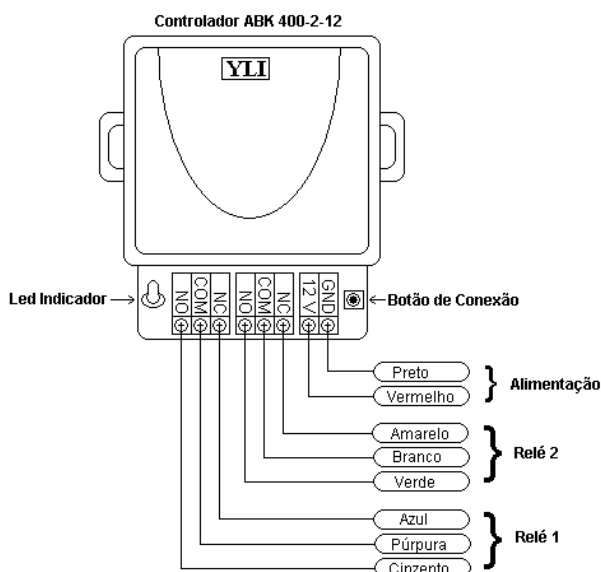
Figura 2. Posição dos dois relés do controlador ABK-400-2-12
